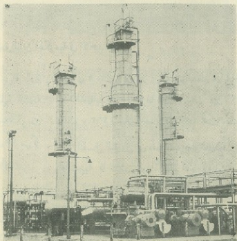
معمل التجزئة لإفاز البترول المسيل في معمل التكرير بالاحمدى
