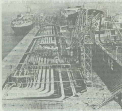
Vista del muelle Ahmadi, considerado como el más largo del mundo, desde el que nace un movimiento de barcos petroleros a todo el mundo.
